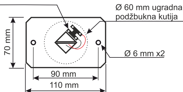
Detalj montaže
